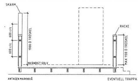
A-A SEKTION GENOM ALTAN
