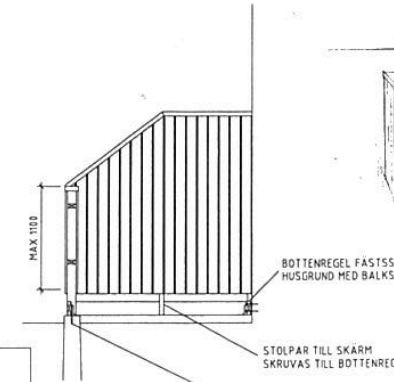
B-B SEKTION GENOM ALTAN
