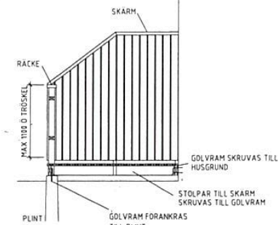
B-B SEKTION GENOM ALTAN
